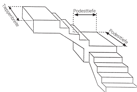
5 Treppe 90° abgewinkelt mit Podest
