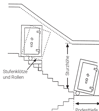
6 Treppe 180° abgewinkelt mit Podest
