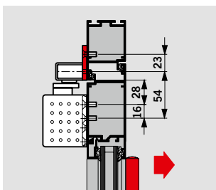
Montageplatte 40 mm für G-N Zur Anbringung der Gleitschiene an Türrahmen, bei denen keine direkte Montage möglich ist.
