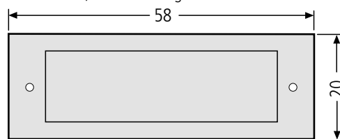
Namensschild ALU-Rahmen eckig EV1 97-9-82192 24,00 € 58 x 20 mm, Verkauf solange Vorrat reicht.
