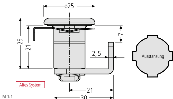
Zylinderschloss ER 97-9-95223 16,10 € Schließung 1-50 inkl. 2 Schlüssel, Einbau ab 2006
