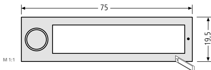
Kunststoff-RSA2-kompakt Namensschildabdeckung ohne Gravur, 97-9-85339 14,90 € für 97-9-85321 und RSA2 -kompakt-Block Seite 11 Einlage max. 59 x 13,6 x 1 mm
