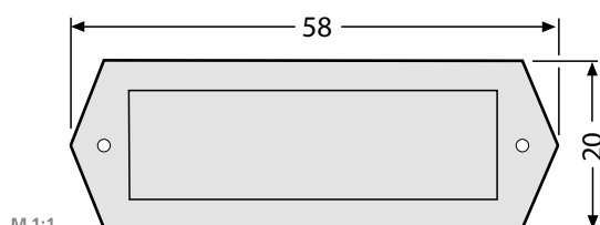
Namensschild ALU-Rahmen EV1 97-9-82186 24,00 € 58 x 20 mm, Verkauf solange Vorrat reicht.
