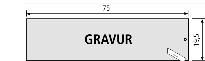
M 1:1 ALU-RSA2 Namensschild 90-3-00028 25,80 € mit schwarzer Gravur* dito Edelstahlausführung 90-3-00027 39,90 € mit weißer Gravur* dito Edelstahlausführung PVD beschichtet 90-3-00033 99,70 € mit weißer Gravur*
