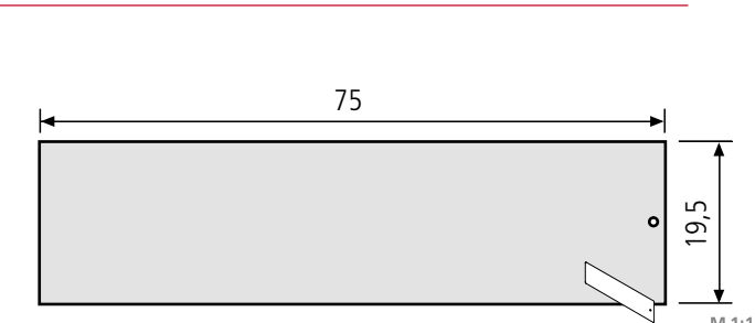
ALU-RSA2 Namensschild ohne Gravur 97-9-85352 14,60 € dito Edelstahlausführung ohne Gravur 97-9-85351 17,50 € dito Edelstahlausführung PVD beschichtet 97-9-85482 77,20 €
