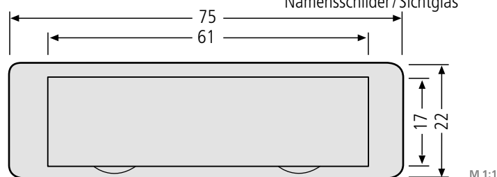
Namensschild 92 – Einbau bis 2009 – 97-9-82016 4,70 € 75 x 22 mm glasklar oder mit grauem Rand (bei Bestellung bitte angeben), Namensschildeinlage max. 60 x 15 x 0,5 mm, Ausstanzung 71 x 19 mm glasklar/0000 oder grau/7039
