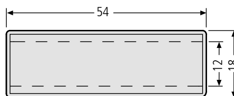
Namensschild – Einbau ab 1970 – 97-9-82014 4,70 € für Durchwurfhals, Namensschildeinlage max. 50 x 12 x 0,5 mm, Ausstanzung 50 x 14 mm
