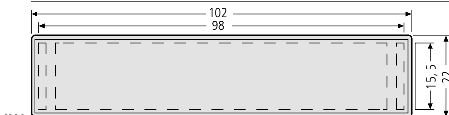
Sichtglas mit Haltekeilen – Einbau ab 1970 – 97-9-82036 4,70 € Ausstanzung 98 x 18 mm
