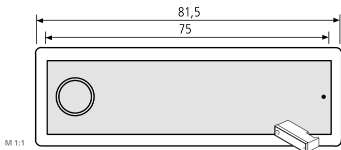
ALU-RSA2-kompakt Klingeltaster 97-9-85319 59,10 €
