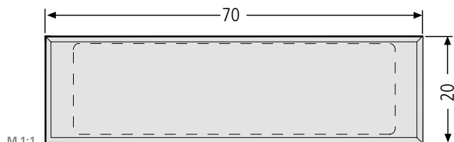
Namensschild 97-9-82173 6,10 € 70 x 20 mm, Ausstanzung 67 x 17 mm. Verkauf solange Vorrat reicht.
