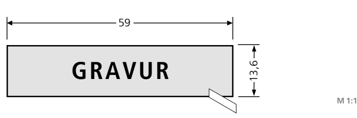
RSA2-kompakt Namensschildabdeckung aus grauem Kunststoff gravierbar, für 97-9-85339, 97-9-85321 u. RSA2 -kompakt-Block Seite 11 ohne Gravur 97-9-87245 3,10 € dito mit Gravur, Schriftfarbe weiß 90-3-00023 14,20 €
