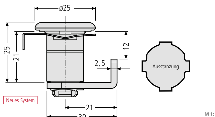
Zylinderschloss ER 97-9-95221 16,10 € Schließung 1-400 inkl. 2 Schlüssel, Einbau ab 2006
