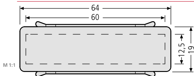
Namensschild 97-9-00303 4,70 € 64 x 19 mm, mit Feder Namensschildeinlage max. 60 x 12,5 x 0,5 mm, Ausstanzung 60 x 15 mm. Einbau für altes Modell: 11-409, 11-410, 12-451, 15-000, 17-200, 17-419, 17-425
