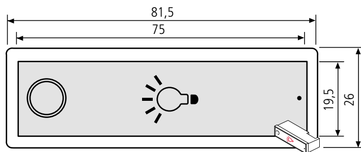
ALU-RSA2-kompakt Lichttaster 97-9-85320 61,00 €
