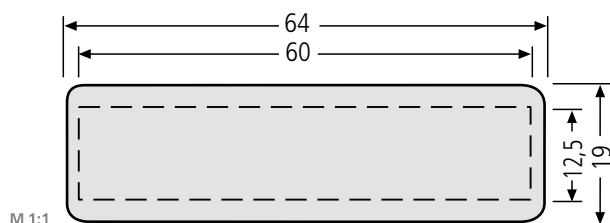
Namensschild – Einbau bis 1978 – 97-9-82019 4,70 € 64 x 19 mm, für 2,5 mm Materialdicke, zum Einklipsen, Namensschildeinlage max. 59,5 x 12,5 x 0,5 mm, Ausstanzung 60 x 15 mm
