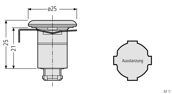
Zylinderschloss ER 97-9-95222 13,90 € Schließung 401-500 inkl. 2 Schlüssel, ohne Riegel Einbau ab 2006
