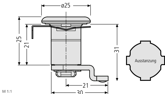
Zylinderschloss ER 97-9-95224 16,10 € Schließung 1-100 inkl. 2 Schlüssel, für Modellgruppe 22 Einbau ab 2006
