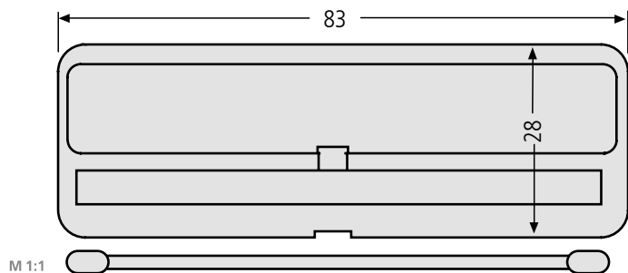
Klappenhalter 97-9-82193 7,10 € mit Torsionsfeder, 83 x 28 mm, Verkauf solange Vorrat reicht.
