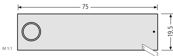
ALU-RSA2-kompakt Namensschild ohne Gravur, 97-9-85338 17,50 € für 97-9-85319 und RSA2 -kompakt-Block Seite 10
