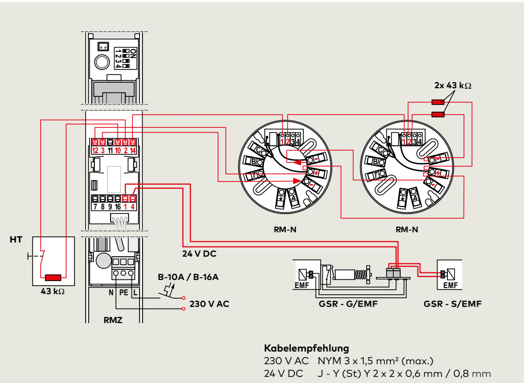
Anschlussplan GSR-EMR XEA mit 2x RM-N
