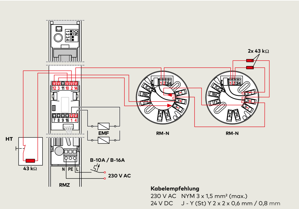
Anschlussplan GSR-EMR XEA mit 2x RM-N
