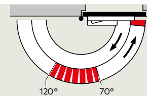
Einstellbare Schliessverzögerung
