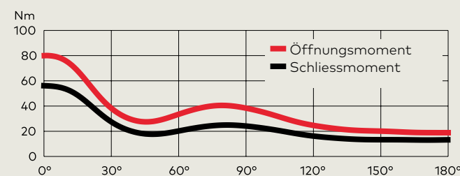
Momentenverlauf TS 98 XEA (Schliesskrafteinstellung EN 6)
