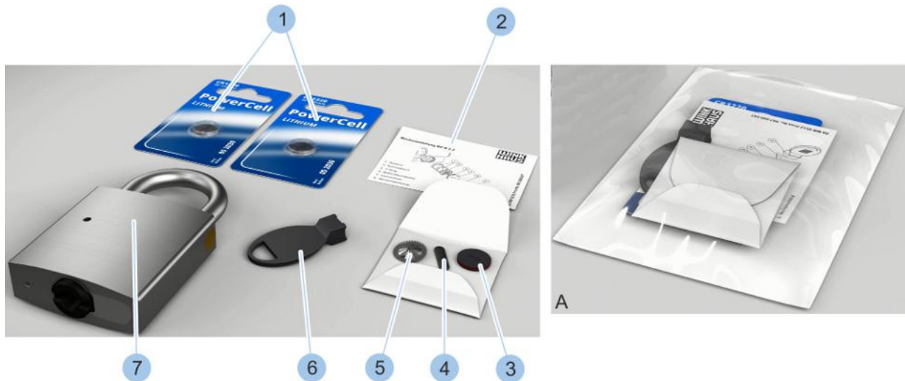
Abb. 99: Batteriewechselset Typ 85
