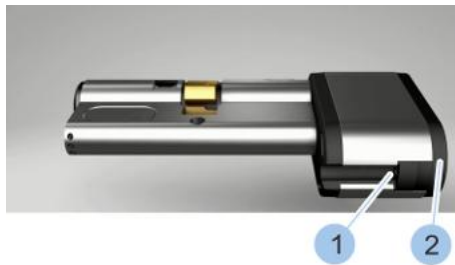
Abb. 98: Batteriefach schließen
