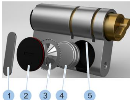
Abb. 104: Batterien wechseln
