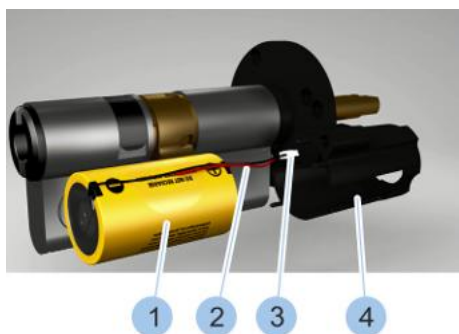
Abb. 90: Batterie entnehmen
