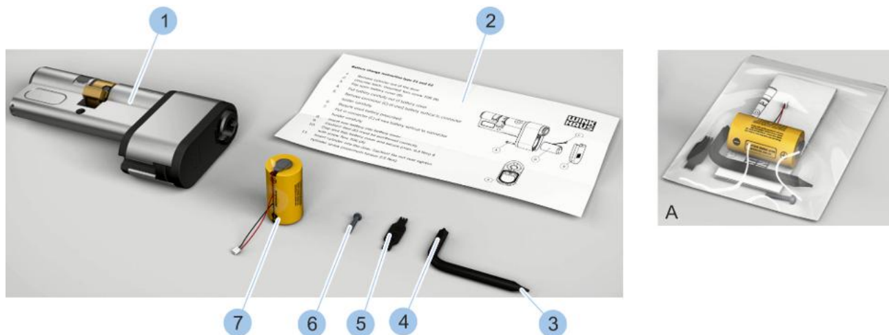
Abb. 94: Batteriewechselset (Typ 21)
