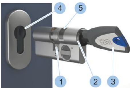
Abb. 32: Zylinder einsetzen
