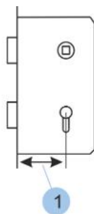
Abb. 30: Dornmaß ausmessen
