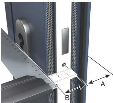
Abb. 26: Zylinder ausmessen
