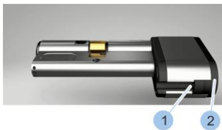
Abb. 95: Batteriefach öffnen
