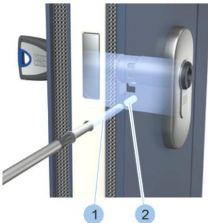
Abb. 34: Stulpschraube einschrauben
