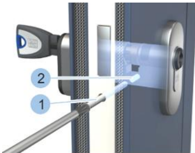
Abb. 42: Zylinder festschrauben
