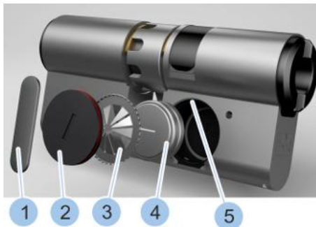
Abb. 83: Batterien einlegen
